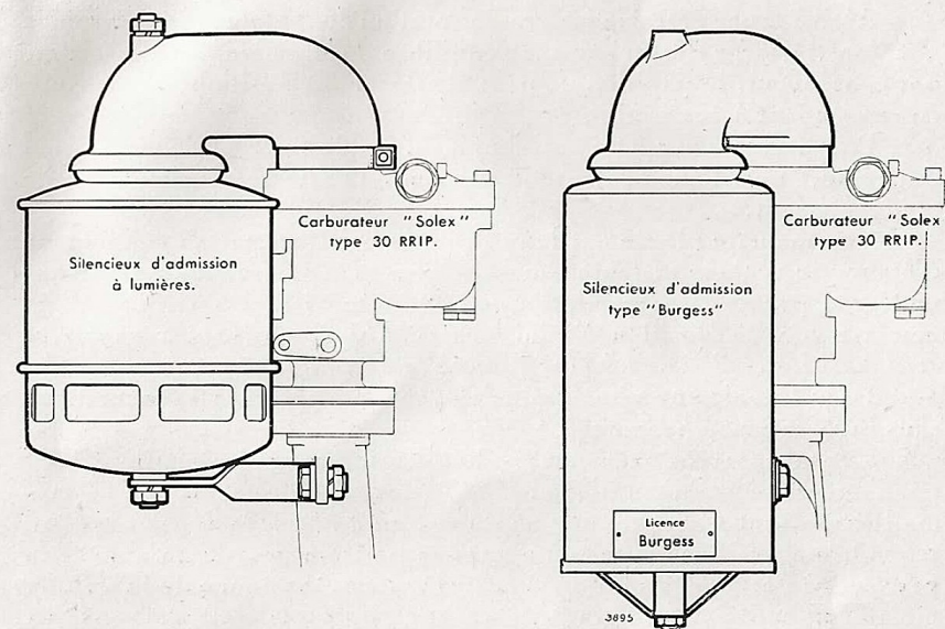
Fig. 17. — Silencieux d'admission.
