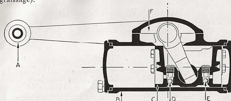
Fig. 13. — Coupe longitudinale.
