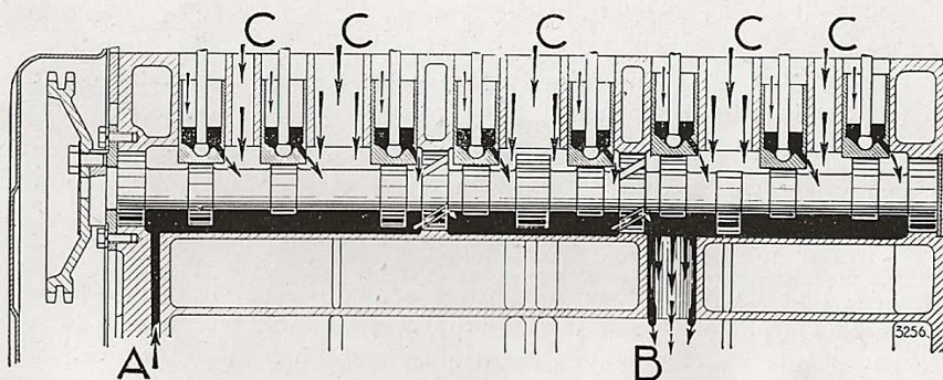
Fig. 28. — Schéma de la circulation d'huile dans le carter d'arbre à cames.
