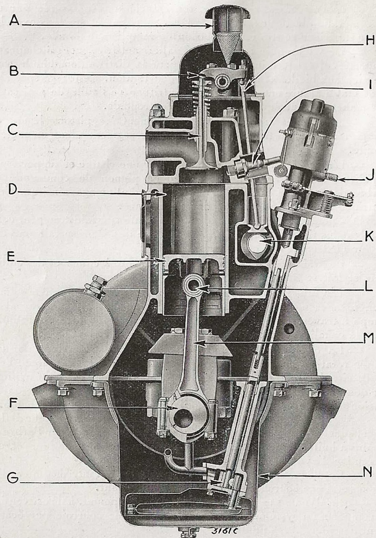
Fig. 7. — Coupe transversale du moteur.
