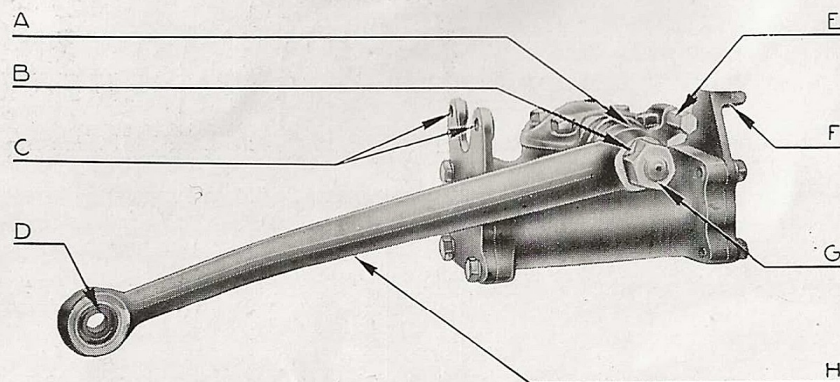
Fig. 12. — Amortisseur hydraulique.
