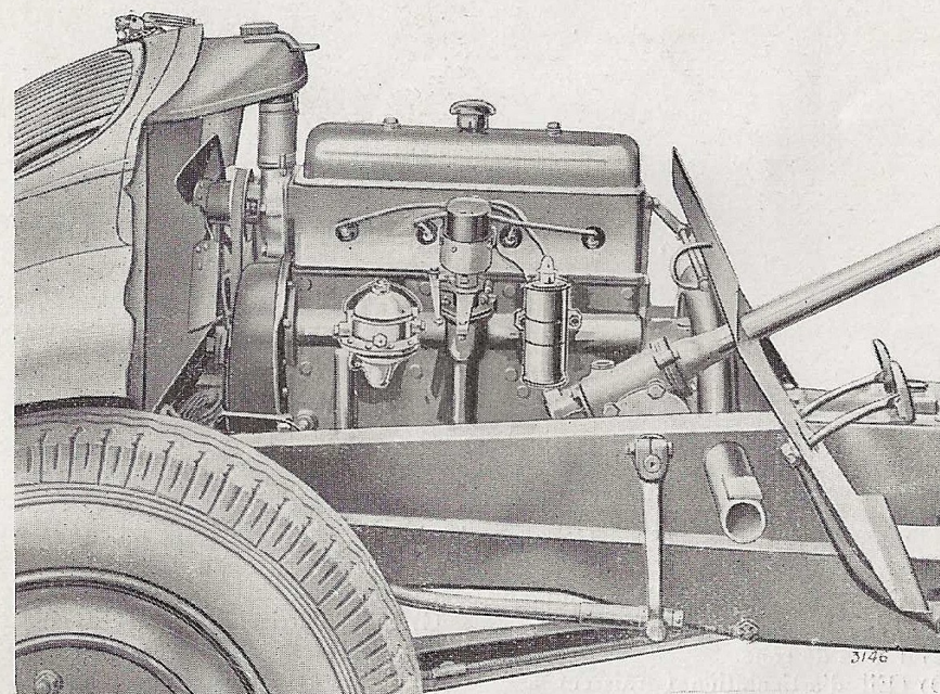
Fig. 4. — Vue latérale gauche du moteur.
