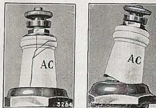
Fig. 39. Cassures provoquées par choc ou mauvaise maintenance.
