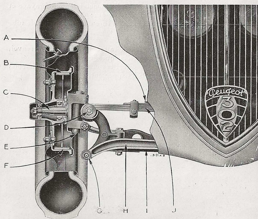
Fig. 5. — Coupe de l'essieu avant droit.
