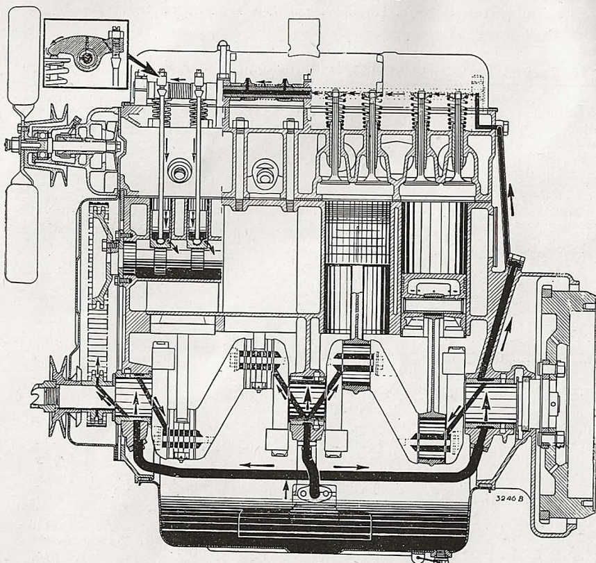
Fig. 27. — Schéma de la circulation d'huile.
