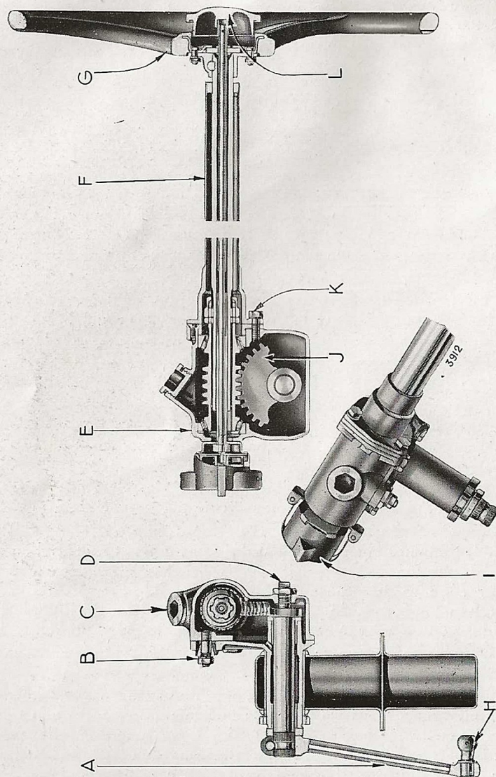
Fig. 21. — Coupe de la direction.
