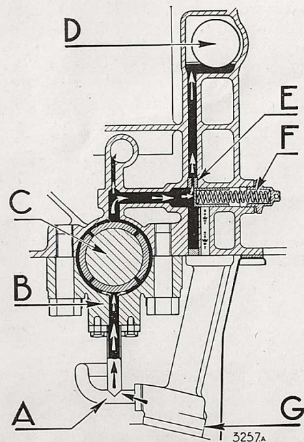
Fig. 26. — Coupe du clapet de décharge. A) Canalisation d'huile. B) Palier avant. C) Vilebrequin. D) Logement de l'arbre à cames. E) Ajustage calibré. F) Ressort du clapet. G) Pompe à huile.
