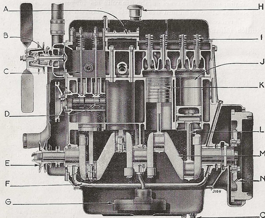
Fig. 6. — Coupe longitudinale du moteur.
