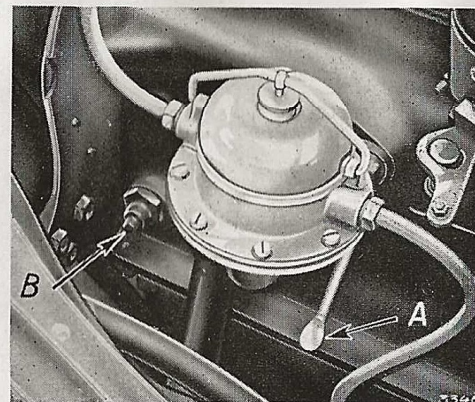
Fig. 18. — Pompe à essence. A) Levier.
