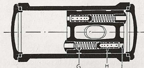
Fig. 14. — Coupe schématique montrant le fonctionnement des amortisseurs.
