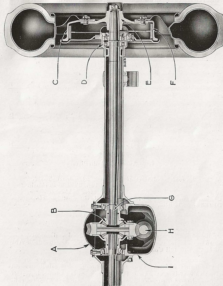
Fig. 11. — Coupe du pont arrière et d'une roue arrière.
