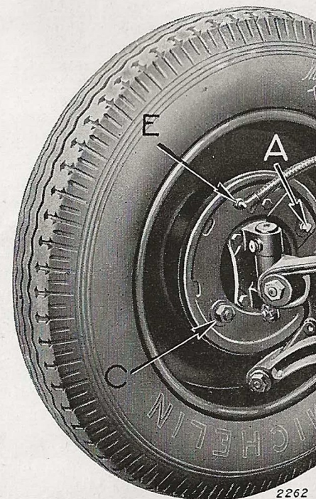
Fig. 22. — Réglage des freins avant.
