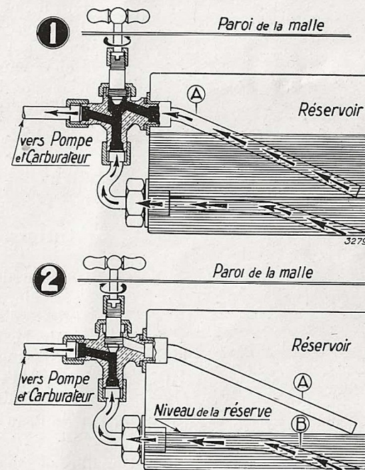
Fig. 43. — Fonctionnement du robinet de réservoir à essence.
