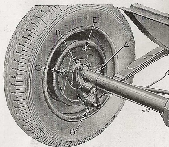
Fig. 23. — Réglage des freins arrière.
