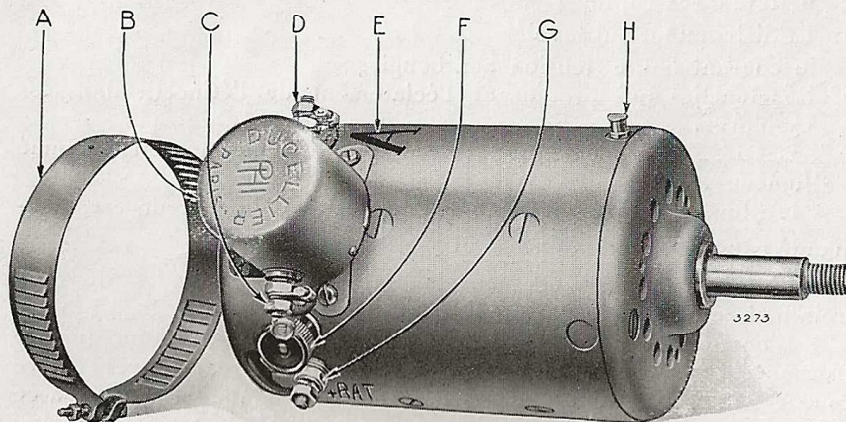
Fig. 40. — Vue de la dynamo anticompond avec sangle démontée.
