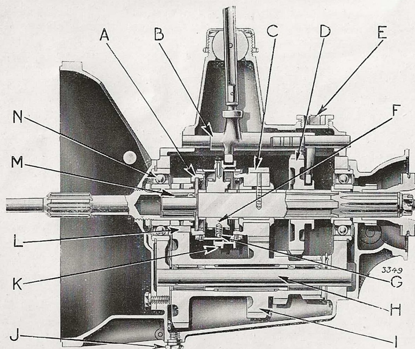
Fig. 9. — Coupe longitudinale de la boîte de vitesses.
