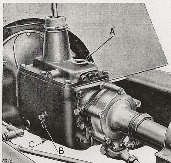
Fig. 29. — Vue de la boîte de vitesses ; A) Bouchon de remplissage. B) Bouchon de niveau, C) Bouchon de vidange.
