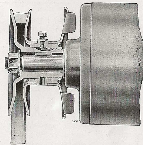
Fig. 19. - Réglage de la courroie de dynamo.
