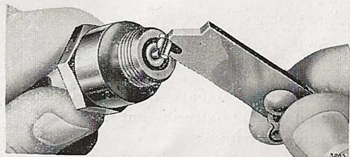
Fig. 38. Outil permettant de régler l'écartement des pointes sans risquer de casser l'isolant.
