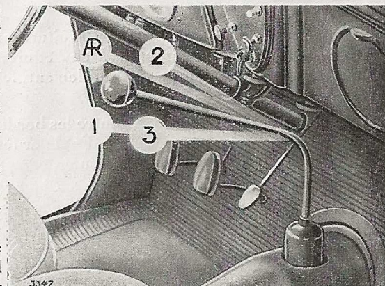
Fig. 42. — Schéma des positions du levier des vitesses.
