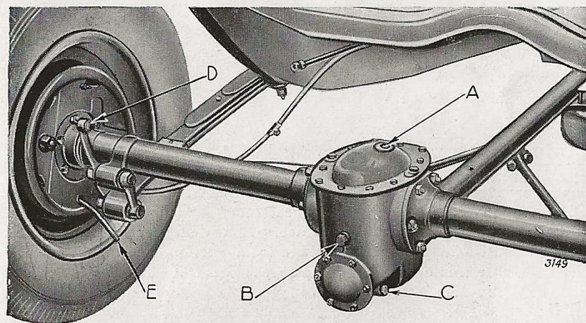
Fig. 30. — Graissage du pont arrière.
